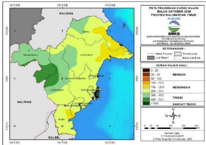
Gambar 25. Peta Prediksi Curah Hujan Oktober 2025
