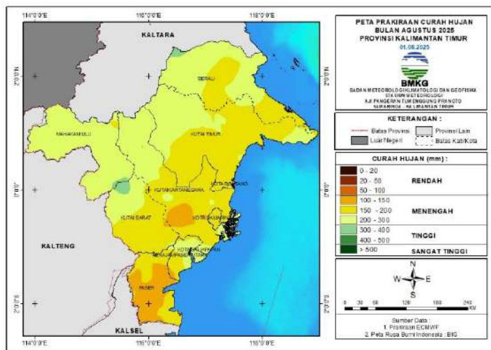
Gambar 21. Peta Prediksi Curah Hujan Agustus 2025
