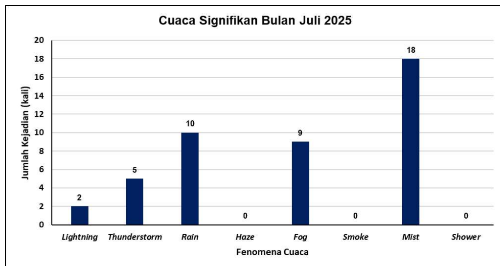
Gambar 13. Grafik Kejadian Cuaca Signifikan Bulan Juli 2025
