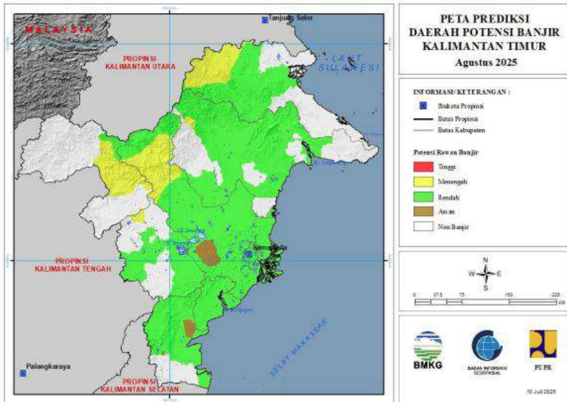
Gambar 27. Peta Prediksi Daerah Potensi Banjir Agustus 2025
