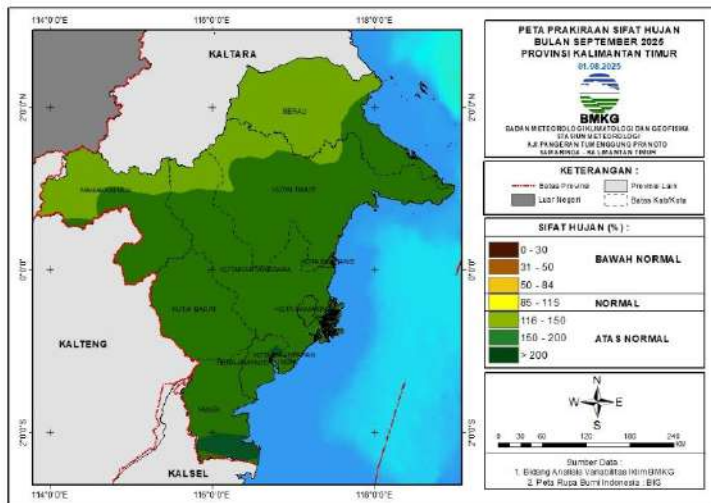
Gambar 24. Peta Prediksi Sifat Hujan September 2025
