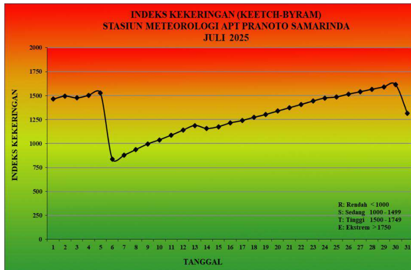
Gambar 14. Grafik Indeks Kekeringan Juli 2025
