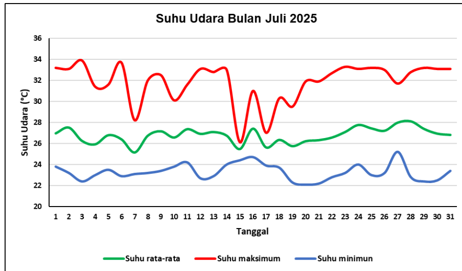
Gambar 9. Grafik Suhu Udara Bulan Juli 2025
