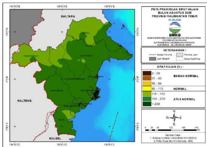
Gambar 22. Peta Prediksi Sifat Hujan Agustus 2025
