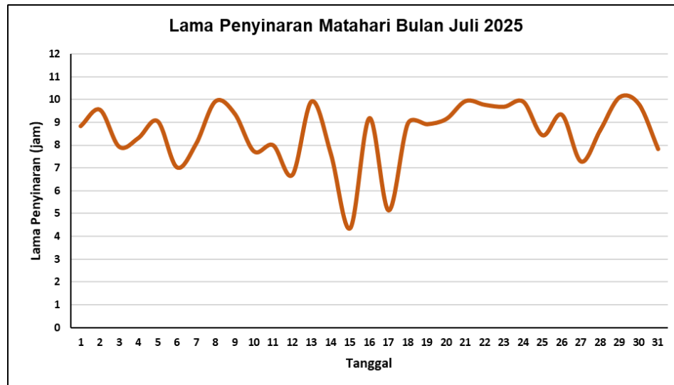
Gambar 11. Grafik Lama Penyinaran Matahari Juli 2025
