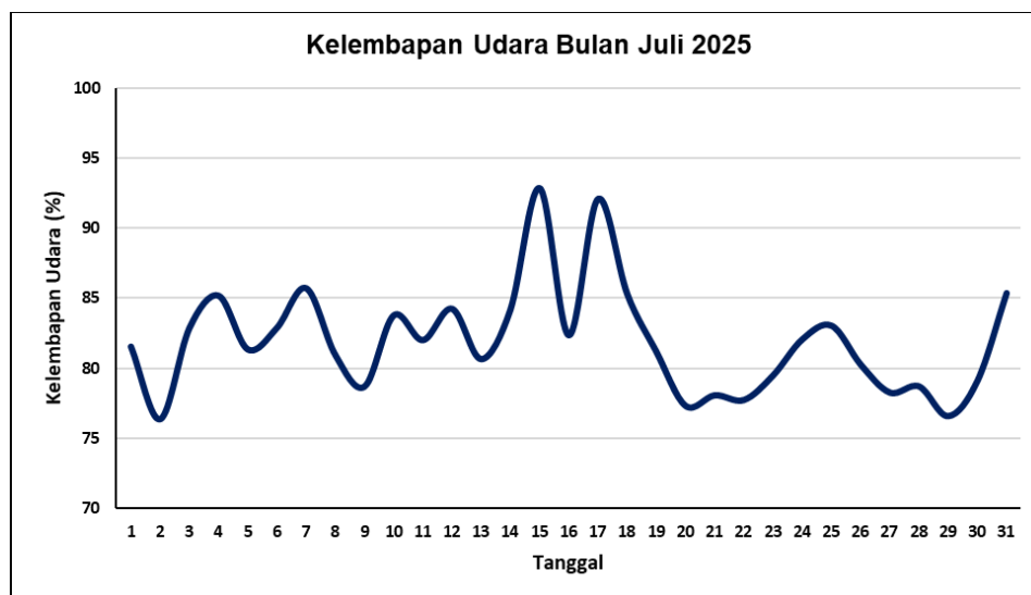
Gambar 10. Grafik Rata-Rata Kelembapan Udara Bulan Juli 2025
