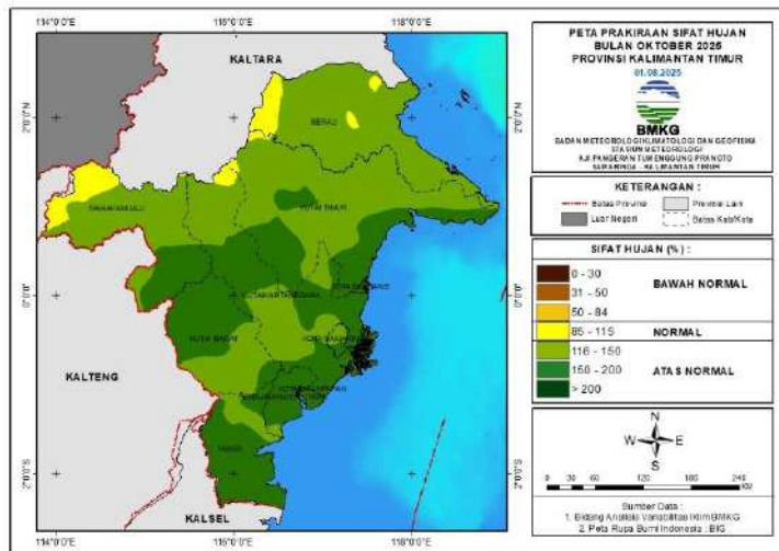
Gambar 26. Peta Prediksi Sifat Hujan Oktober 2025
