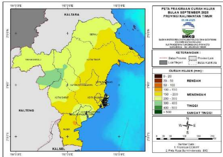
Gambar 23. Peta Prediksi Curah Hujan September 2025
