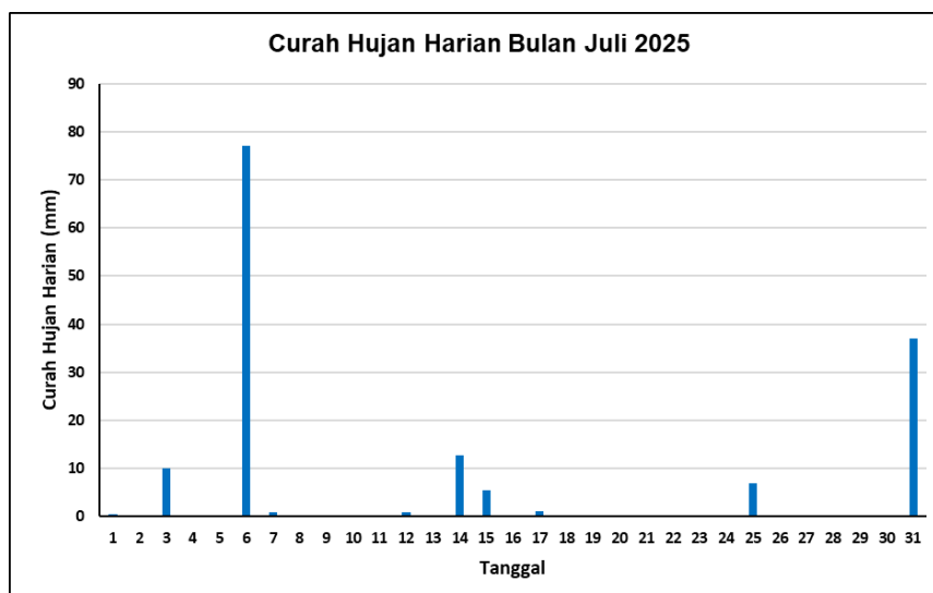
Gambar 8. Grafik Curah Hujan Harian Bulan Juli 2025
