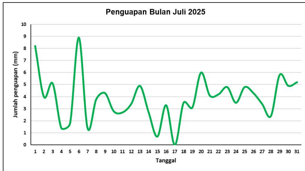
Gambar 12. Grafik Penguapan Bulan Juli 2025
