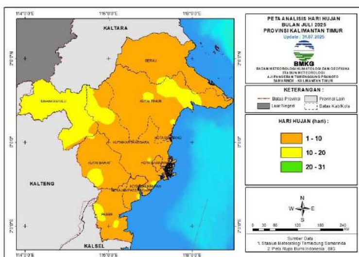
Gambar 20. Peta Analisis Hari Hujan Juli 2025
