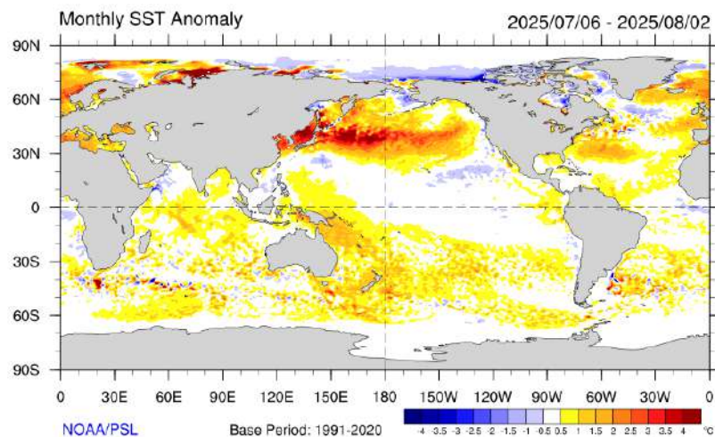
Gambar 5. Peta Anomali SST Juli 2025
