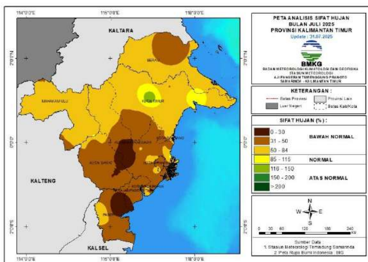
Gambar 19. Peta Analisis Sifat Hujan Juli 2025
