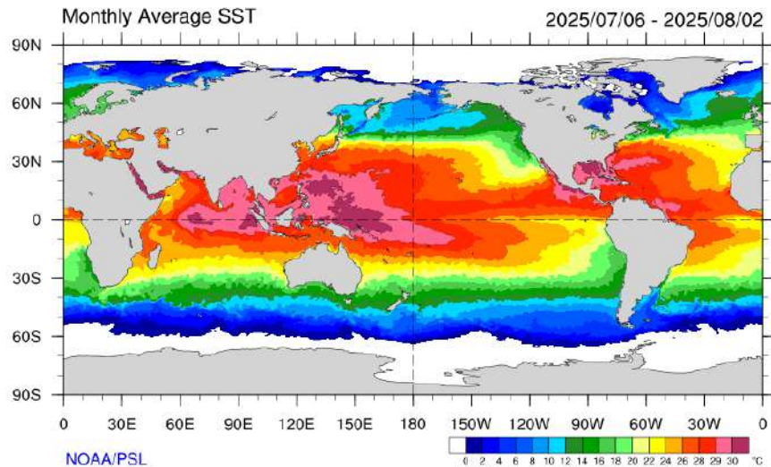
Gambar 4. Peta SST Juli 2025
