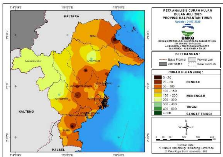
Gambar 18. Peta Analisis Curah Hujan Juli 2025
